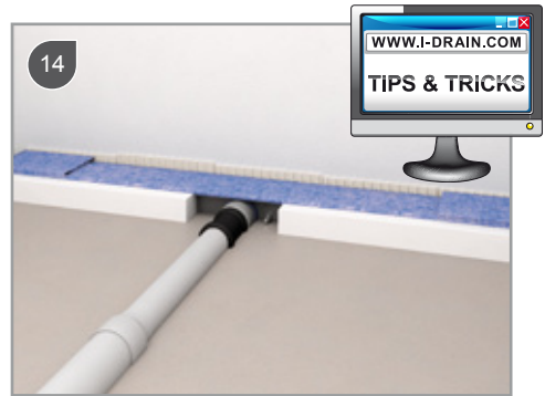
14 Specievloer aanbrengen afhellend (1 – 2%) naar de drain toe / Apply the screed with a fall (1 – 2%) towards the drain / Faire la chape avec une pente (1 - 2%) en direction du drain / Estrich mit Gefälle von 1% - 2% zur Rinne einbauen
