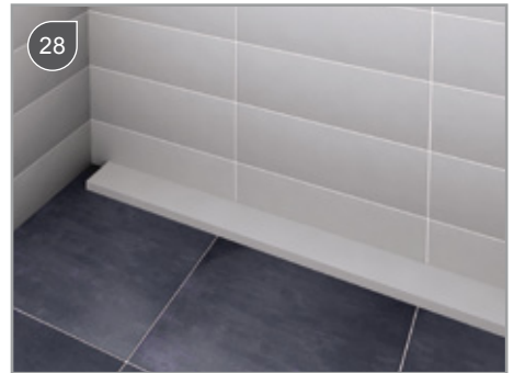
28 Vloertegels plaatsen / Fixation of the floor tiles / Poser le carrelage au sol contre le guide de pose en polystyrène / Bodenfliesen bis an das Styropor Rinnen Innenteil ankleben
