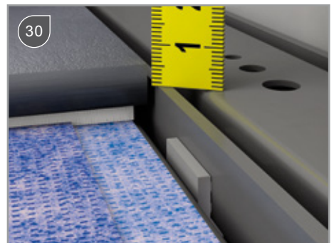
30 Bereken het aantal benodigde verhogingsblokjes / Calculate the required number of rising blocks / Déterminer le nombre de blocs de rehausse nécessaire / Berechnen Sie das erforderliche Zahl Rosterhöhungsstücke
