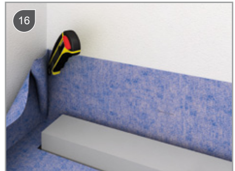
16 Uitsnijden van het hoekdeel in de waterdichtingsmat / Cutting out the corner part in the waterproofing mat / Découper le tapis imperméable au niveau des coins / Das Eck aus dem Dichtungsvlies ausschneiden
